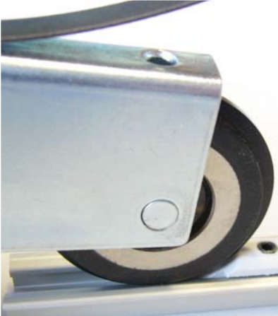
Bodenschiene: einläufig
